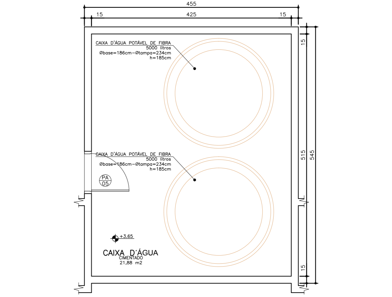
Planta Borda Caixa D'água Esc: 1:50
