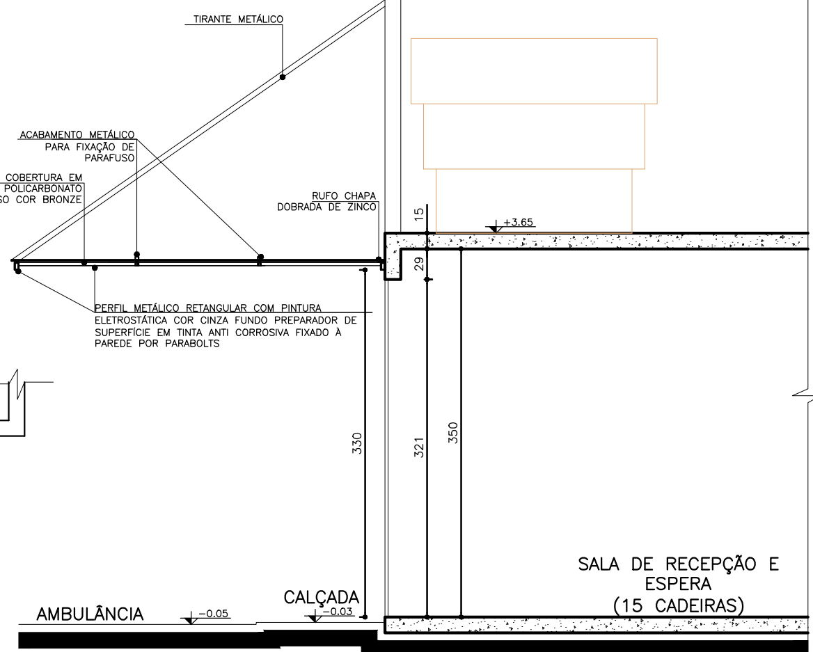
03 Seção A A'-Marquise Entrada Principal Esc.: 1:50
